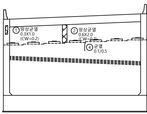
정 면 도
